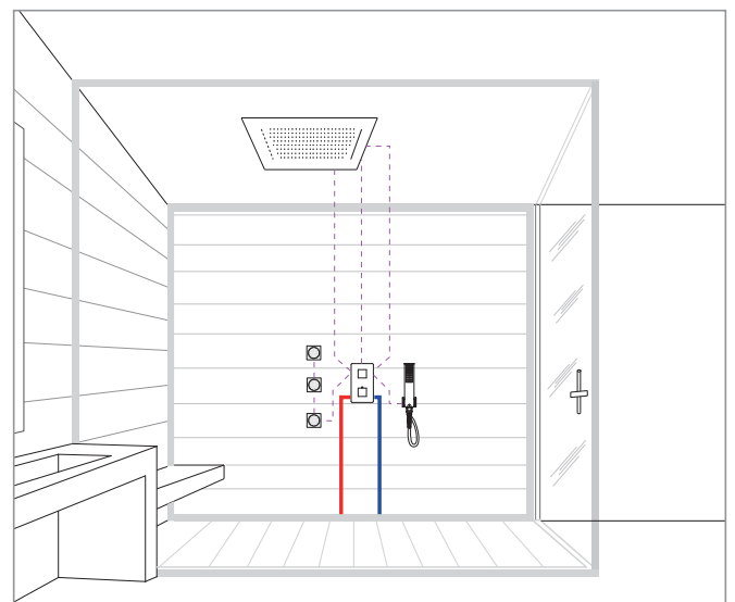
5 WAYS 5 USCITE 5 OUTLETS
