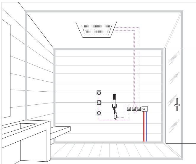
5 5 USCITE: 2 deviatori con 2 vie + 1 via singola WAYS 5 OUTLETS: Nr. 2 2-ways diverters + 1 single way
