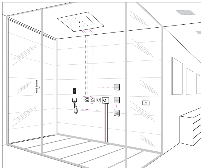
6 6 USCITE: 3 deviatori con 6 vie WAYS 6 OUTLETS: Nr. 3 2-ways diverters
